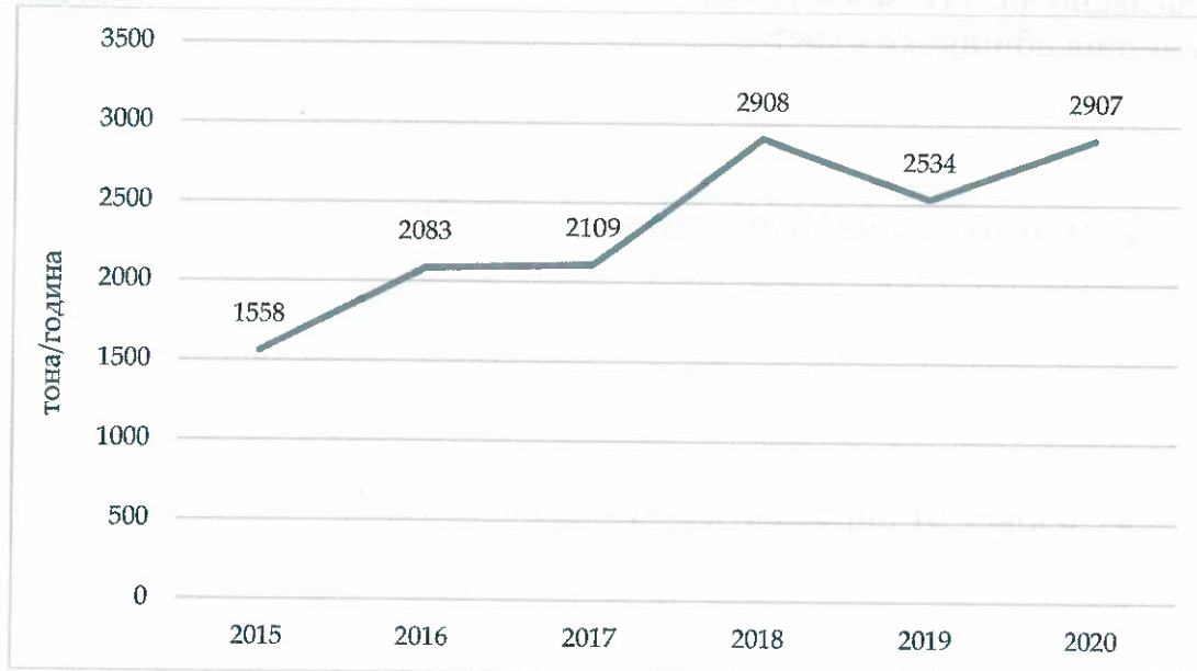
Фигура 3 Произведена електроенергия (MWh) в инсталация за биологично третиране „Хан Богров“
