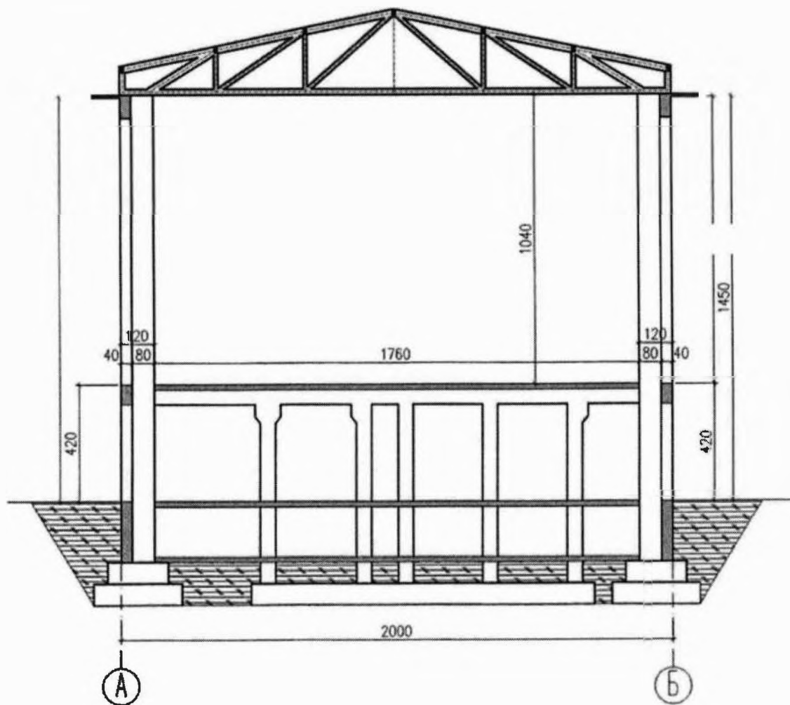
Вертикален разрез:
